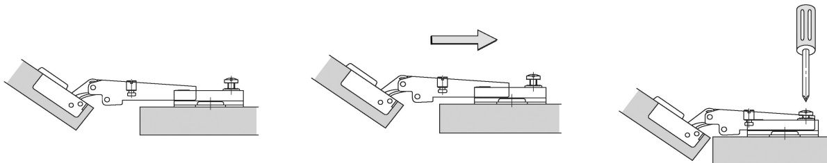
Mounting plate fixed with wood screws Plaque de montage à l'aide de vis à bois
